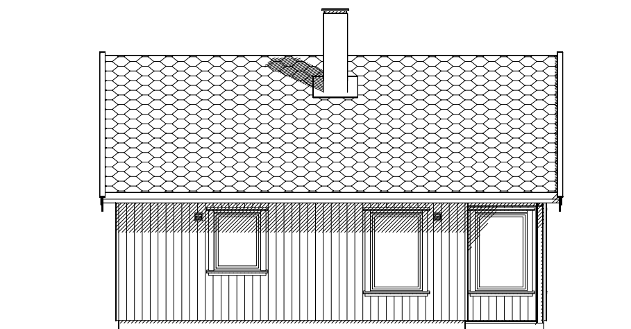
Fasade - 4
