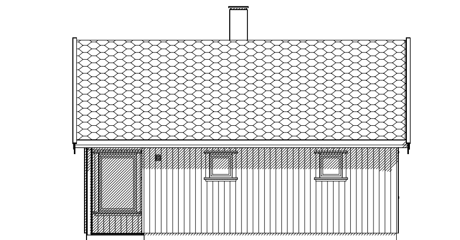
Fasade - 2
